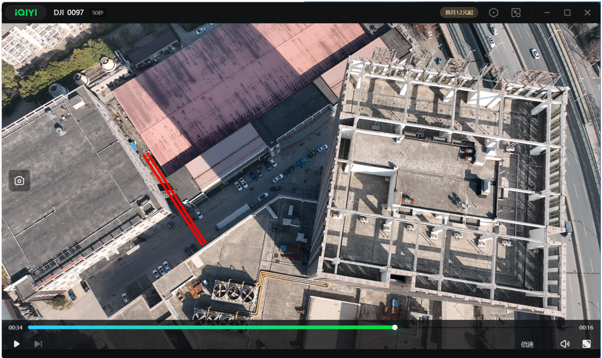
红色区域部分需加装喷淋水系统，加装镀锌钢管DN150，约87m
